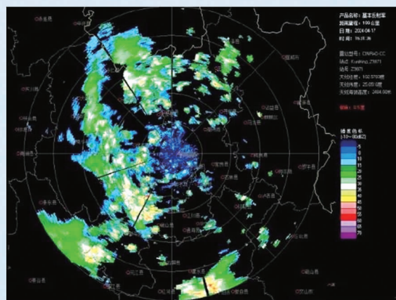
昆明市气象台发布的昆明站雷达图
